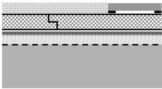
Figuur 2 – Omgekeerd daksysteem op bestaande warmdakconstructie (renovatie)
