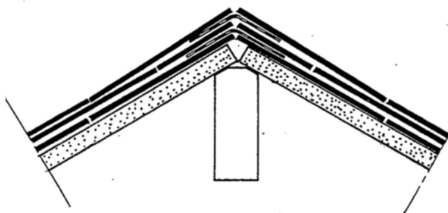
Detail 6a. Hoekkeperaansluiting
