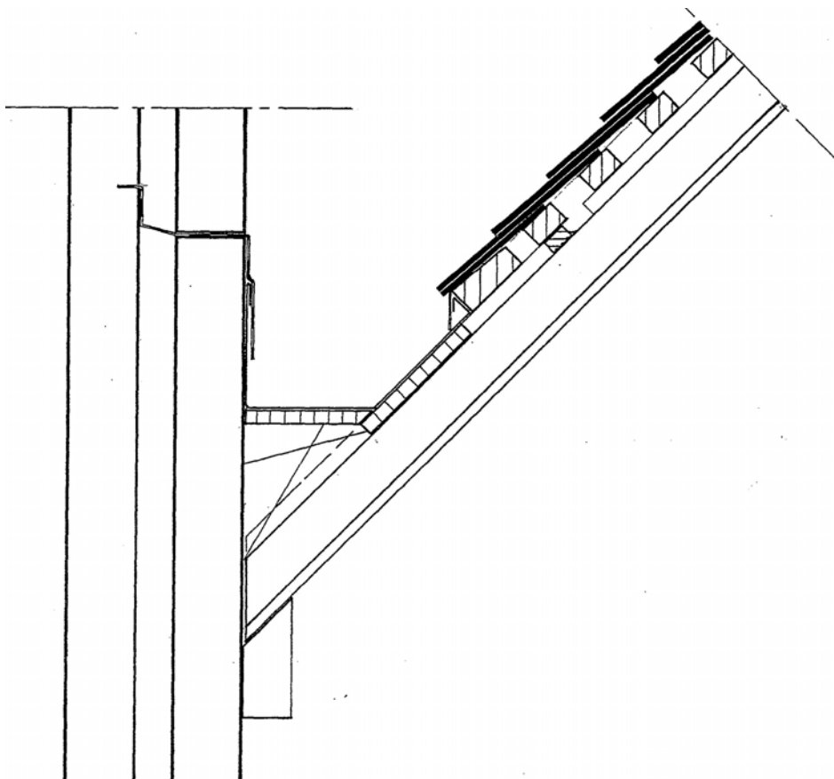
Detail 10a. Bovenaansluiting schoorsteen
