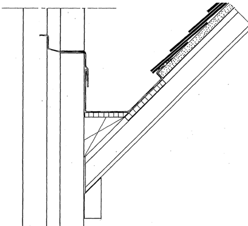
Bovenaansluiting schoorsteen
