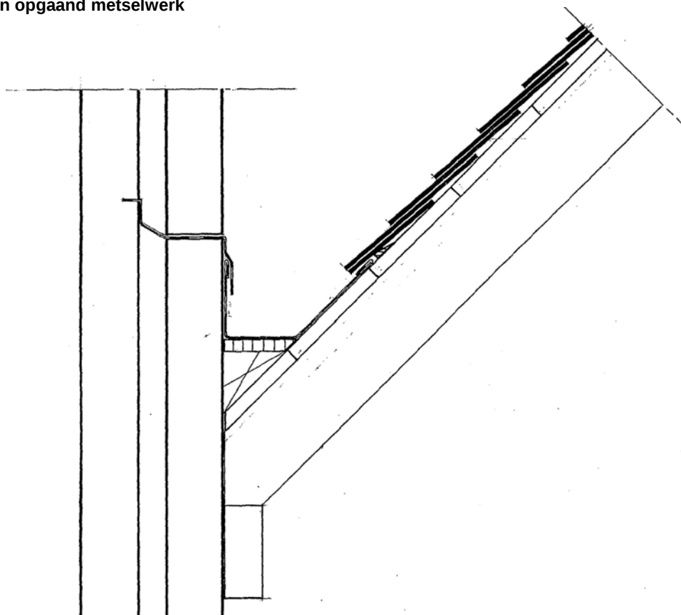
Detail 10a. Bovenaansluiting schoorsteen
