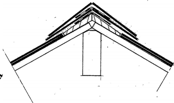
Detail 6d. Hoekkeperaansluiting
