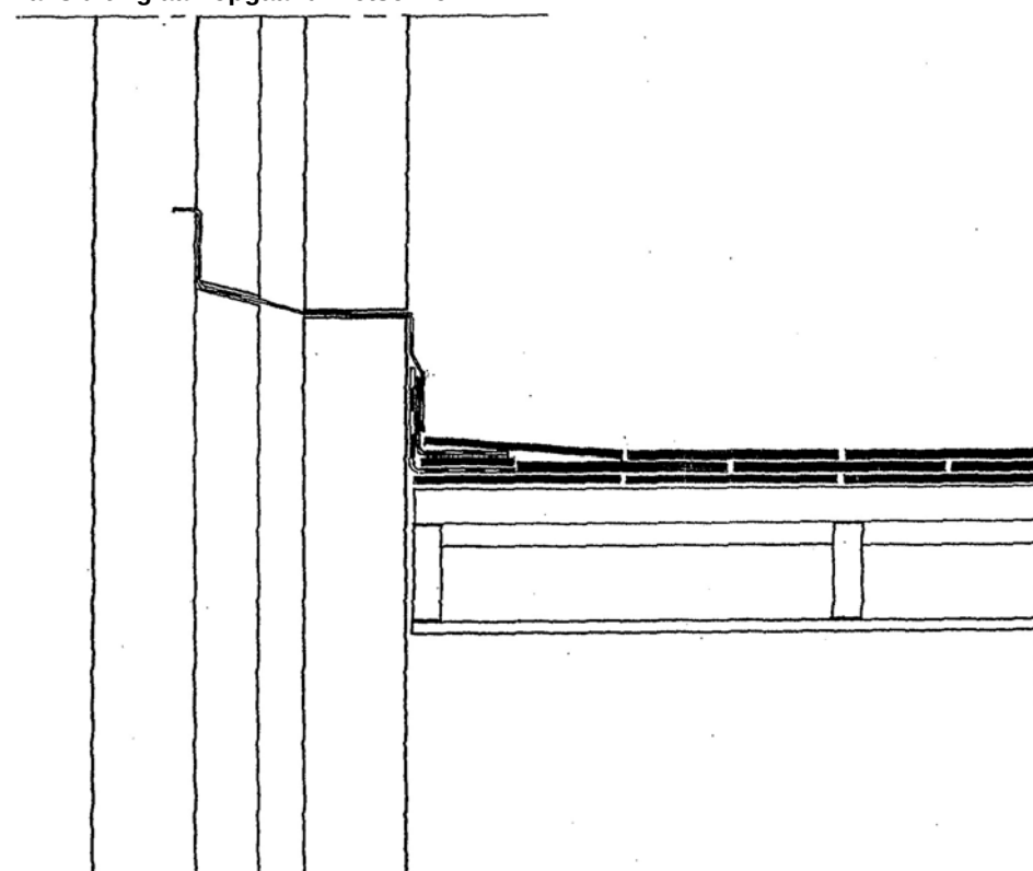
Detail 9a. Aansluiting aan opgaand metselwerk
