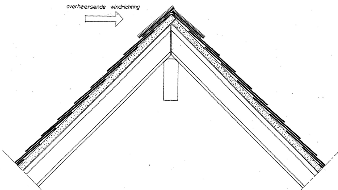
Detail 3d. Nokaansluiting
