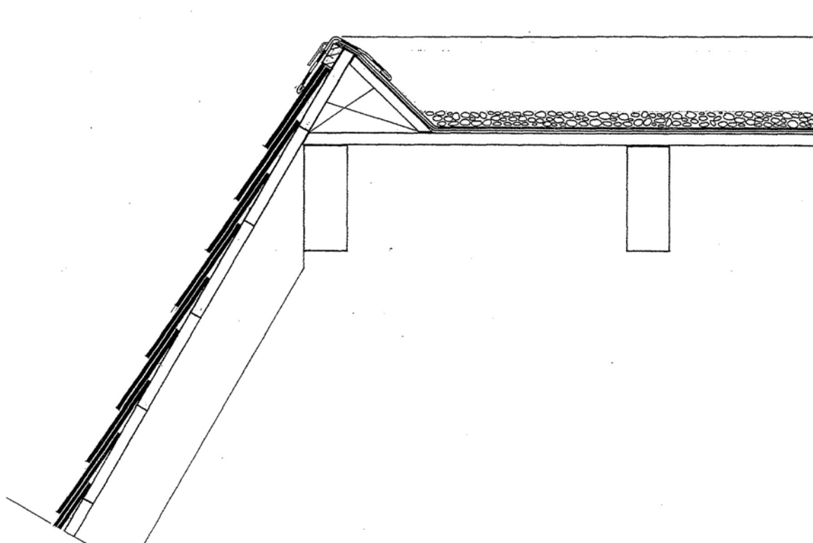
Detail 5a. Nokaansluiting aan plat dak
