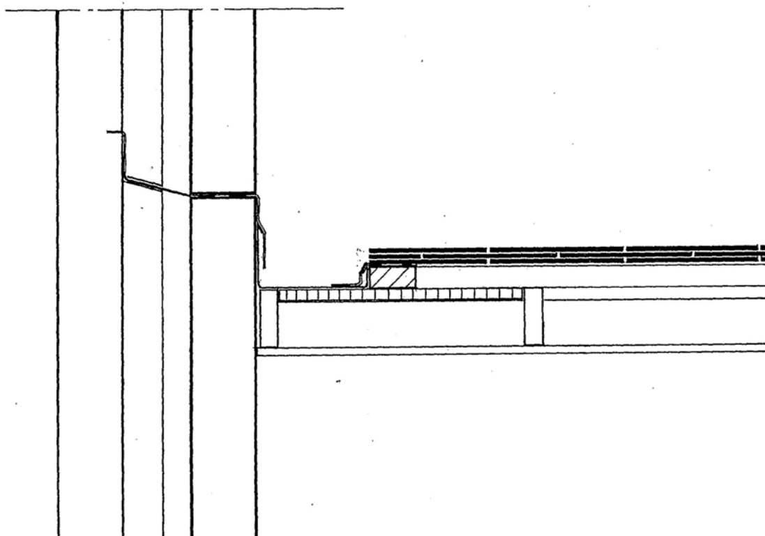
Detail 9a. Aansluiting aan opgaand metselwerk
