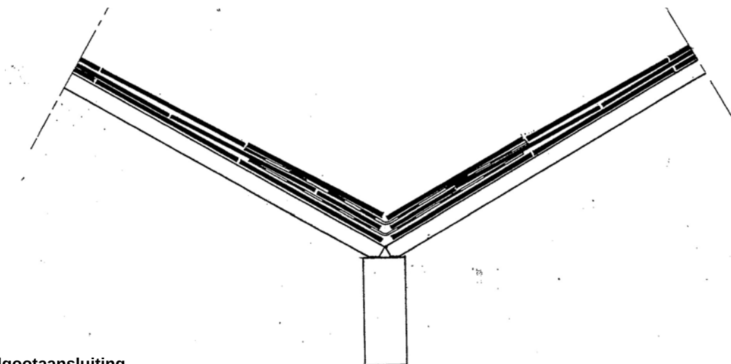
Detail 8a. Kilgootaansluiting
