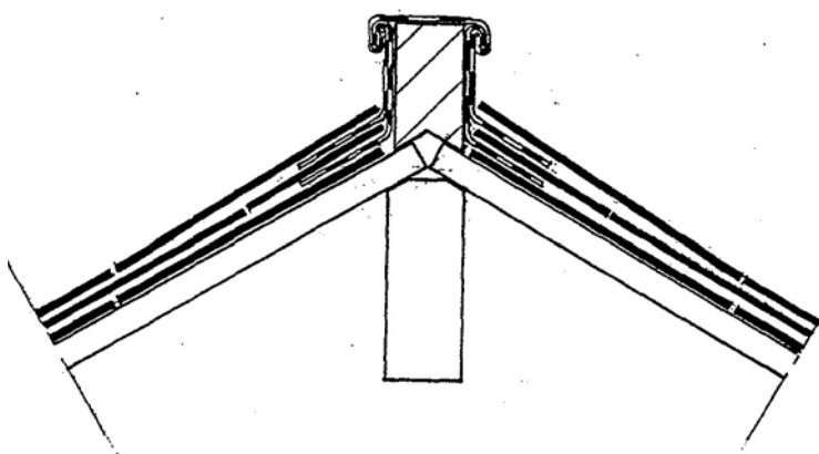
Detail 6c. Hoekkeperaansluiting
