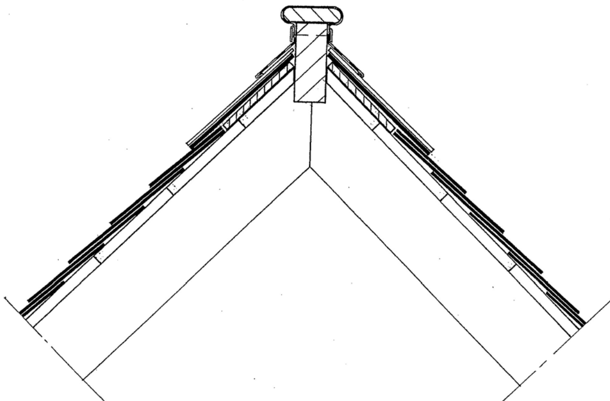
Detail 3c. Nokaansluiting
