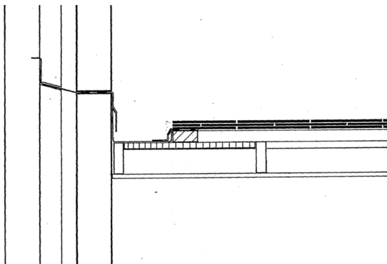
Detail 9c. Aansluiting aan opgaand metselwerk
