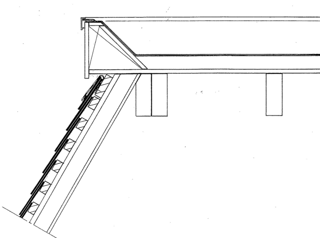
Detail 5a. Nokaansluiting aan plat dak
