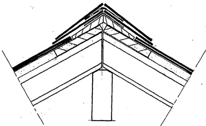
Detail 6c. Hoekkeperaansluiting
