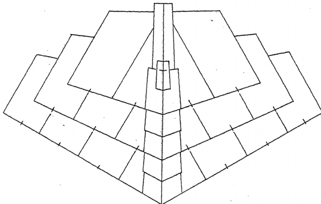
Detail 6f. Hoekkeperaansluiting
