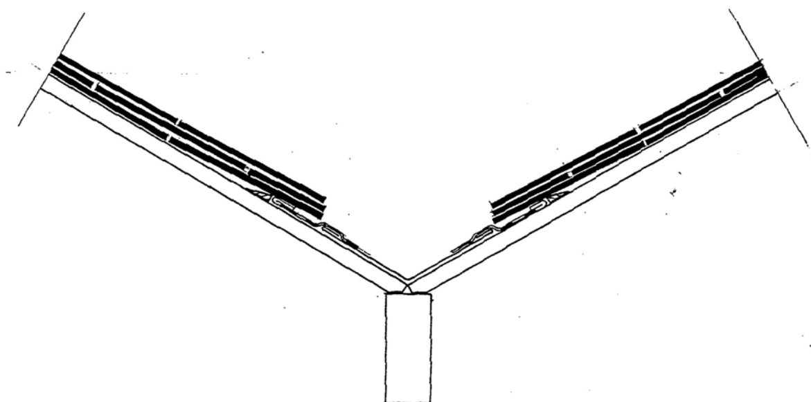
Detail 8c. Kilgootaansluiting
