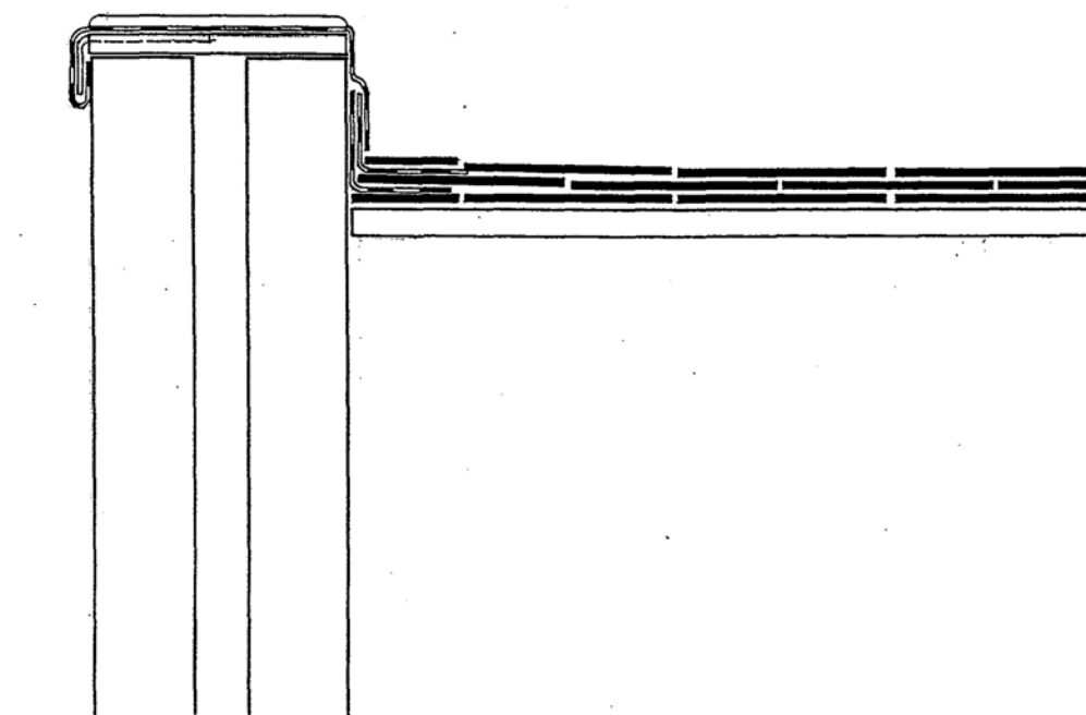
Detail 7a. Aansluiting kopgevel
