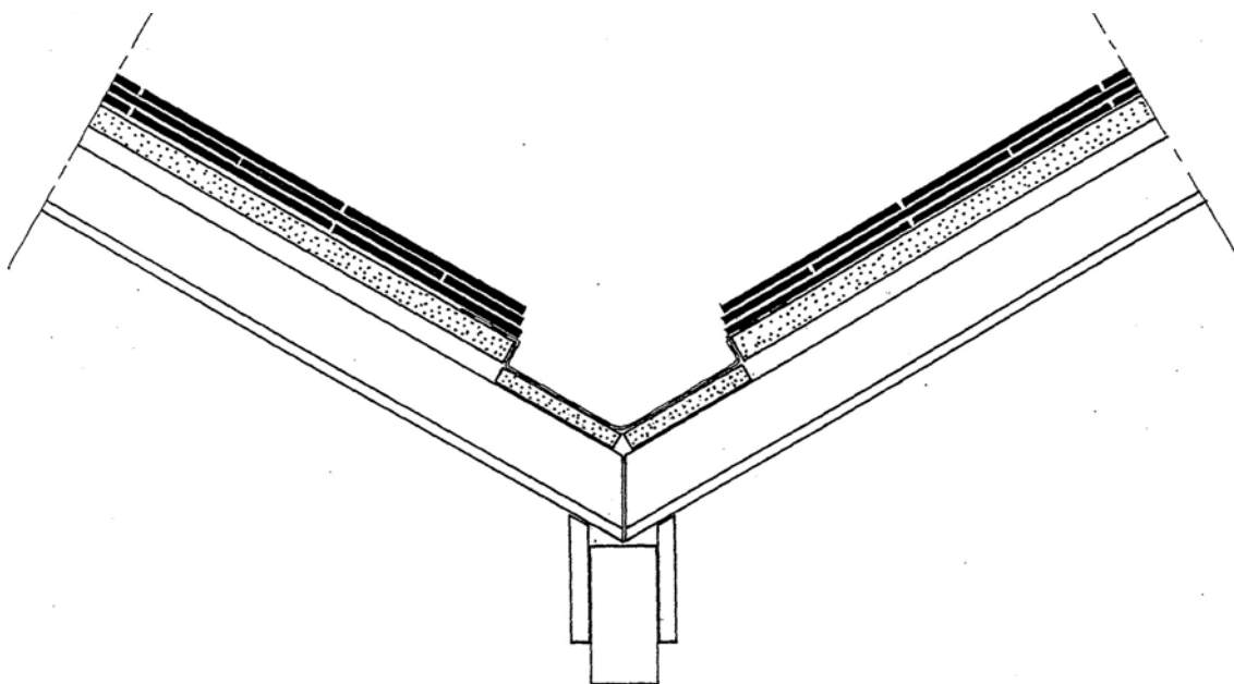
Detail 8d. Kilgootaansluiting
