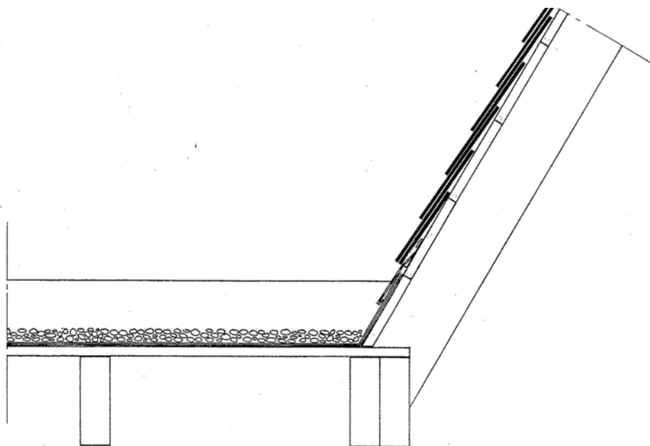
Detail 2a. Dakvoetaansluiting aan plat dak
