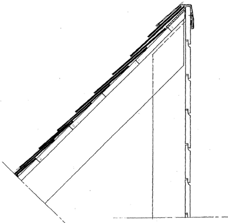
Detail 4a. Nokaansluiting lessenaarsdak
