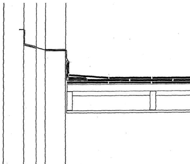
Detail 9d. Aansluiting aan opgaand metselwerk
