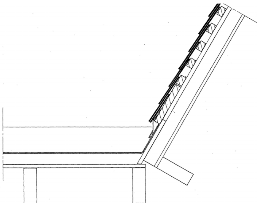
Detail 2a. Dakvoetaansluiting aan plat dak
