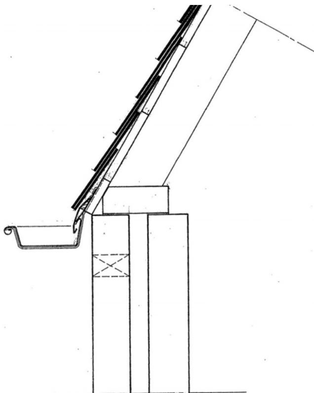
Detail 1c Dakvoetaansluiting
