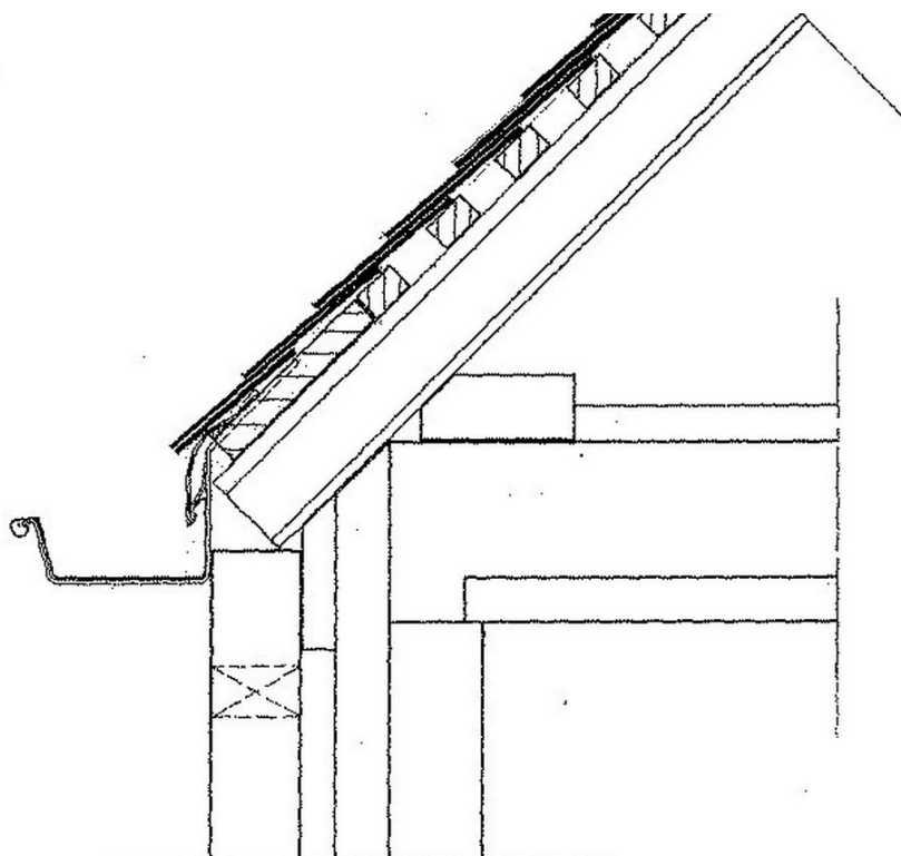
Detail 1b Dakvoetaansluiting
