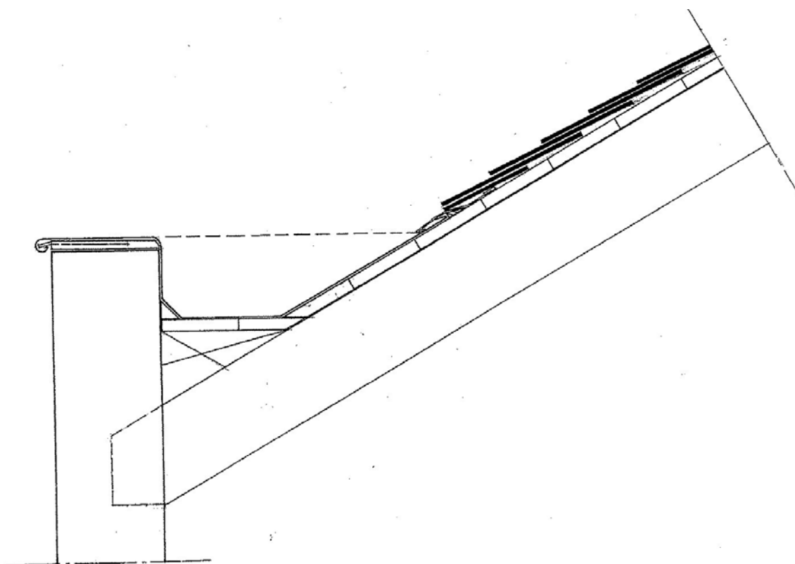
Detail 1g. Dakvoetaansluiting
