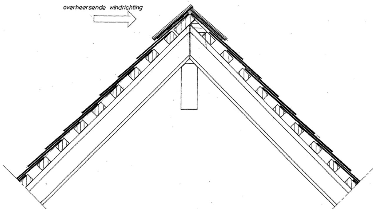
Detail 3a. Nokaansluiting
