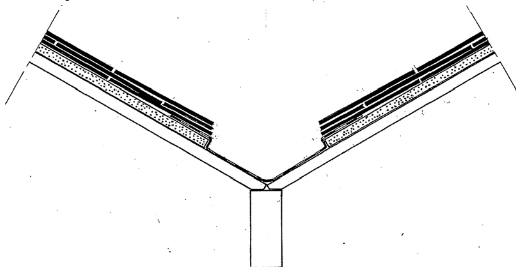
Detail 8b. Kilgootaansluiting
