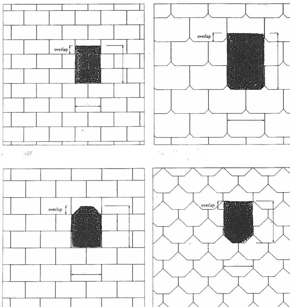
Figuur 8. Formaten en dekkingspatronen Maasdekking
