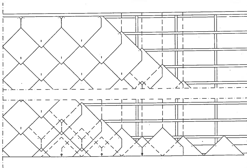
Figuren 17, 18 en 19. Versneden lei en montage ruitdekking
