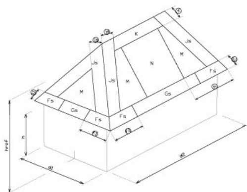
3. Vierzijdig zadeldak
