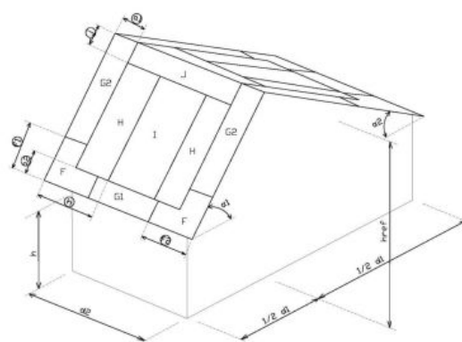
4. Ongelijkzijdig zadeldak
