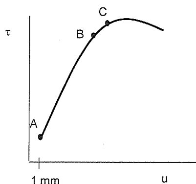
Figuur 5. Spanning-verplaatsings-diagram
