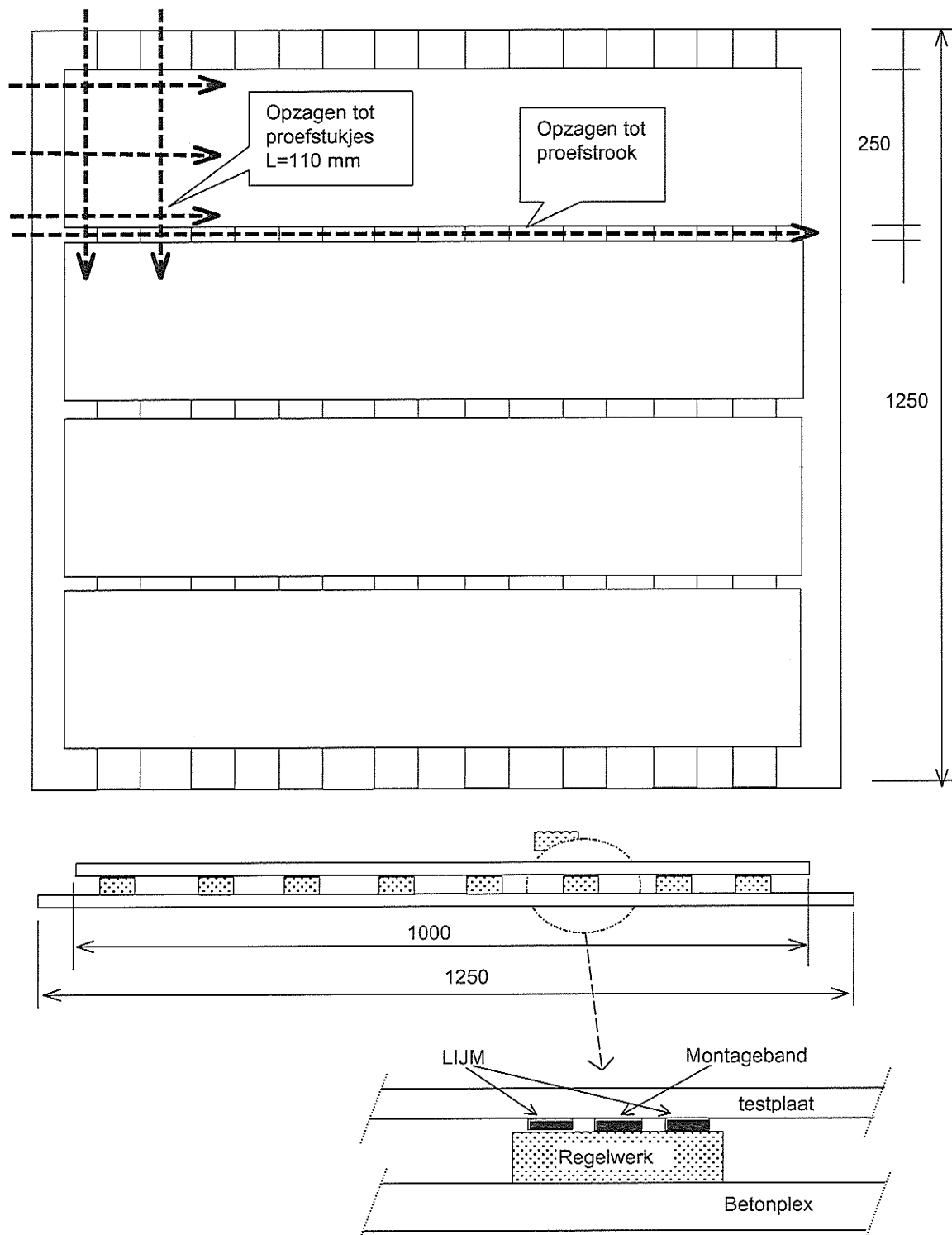
Figuur 3: Opbouw proefplaat t.b.v. deelonderzoek 1 en 2
